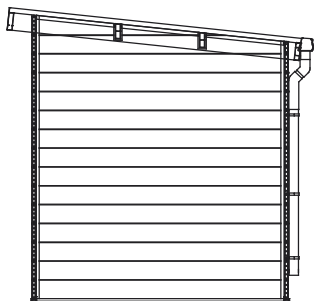
NL ZIJAAANZICHT FR VUE LATÉRALE EN SIDE VIEW DE SEITENANSICHT
